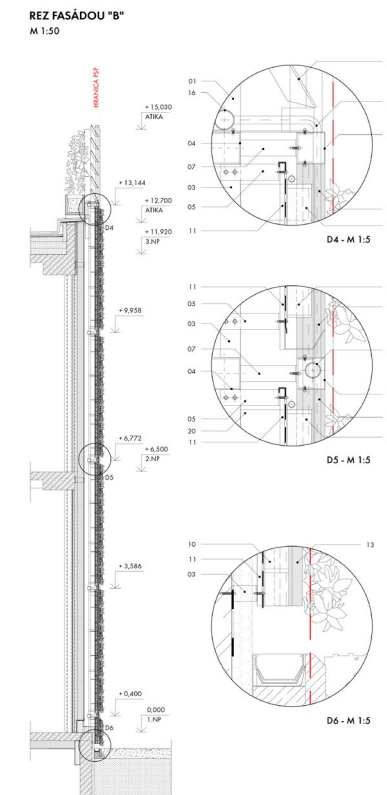
Řez fasádou
