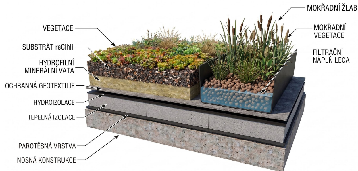
Řez hybridní zelenou střechou. Obrázek vytvořen AI, poskytnut autorem textu.
