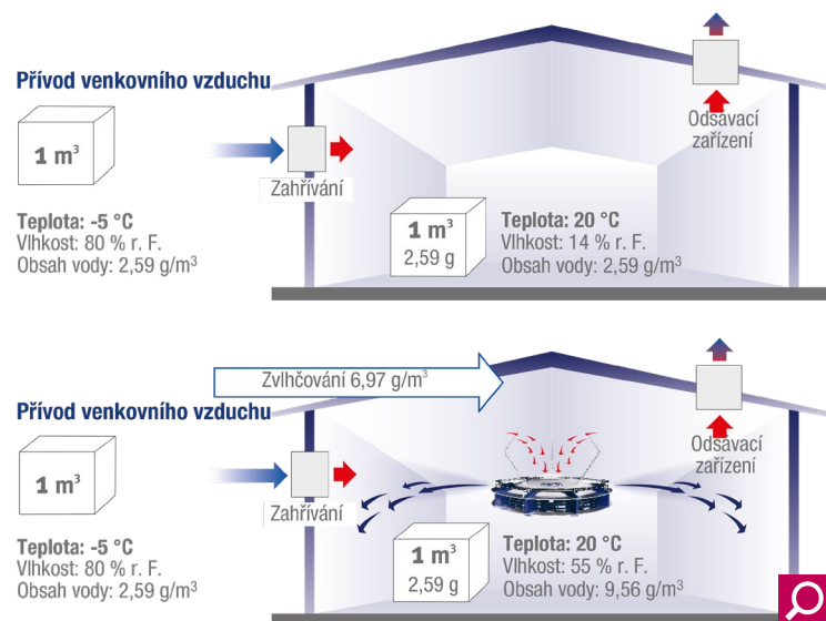
Schéma zvlhčování – porovnání prostor bez destratifikátoru a s destratifikátorem
