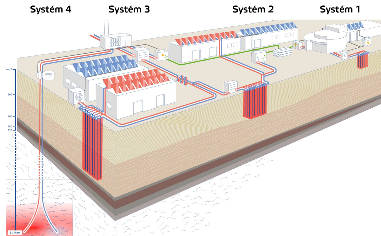
Systém 1 – Zelená budova, systém 2 – Zelený vodík, systém 3 – Mělké zelené teplo, systém 4 – Hluboké zelené teplo
