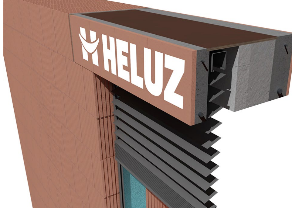
Překlad HELUZ 3in1 nosný pro stínící techniku
