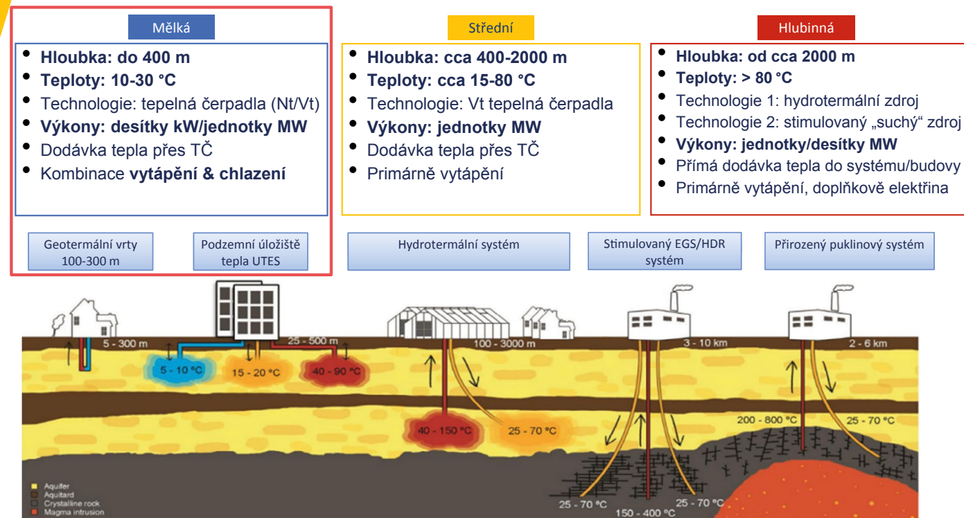
Geotermální energie – klasifikace (Zdroj: Synergys)
